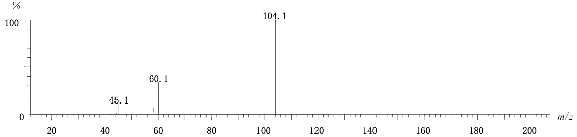
图 B.1 胆碱标准品(100 \mu\text{g/L} )质谱扫描图
