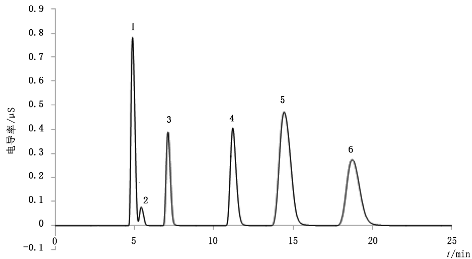
图 A.1 IonPac CS12A 色谱柱等度淋洗色谱图(胆碱标准溶液浓度 1 mg/L)
