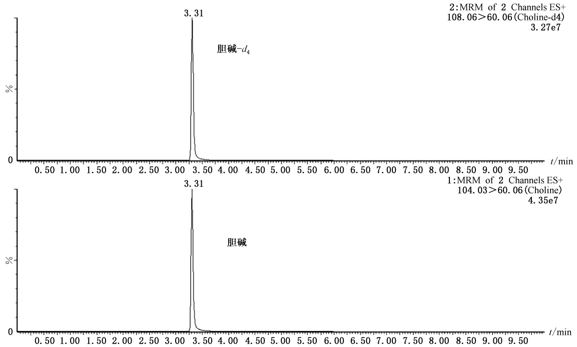
图 B.2 胆碱标准溶液(50 \mu\text{g/L} )及其内标的 MRM 图
